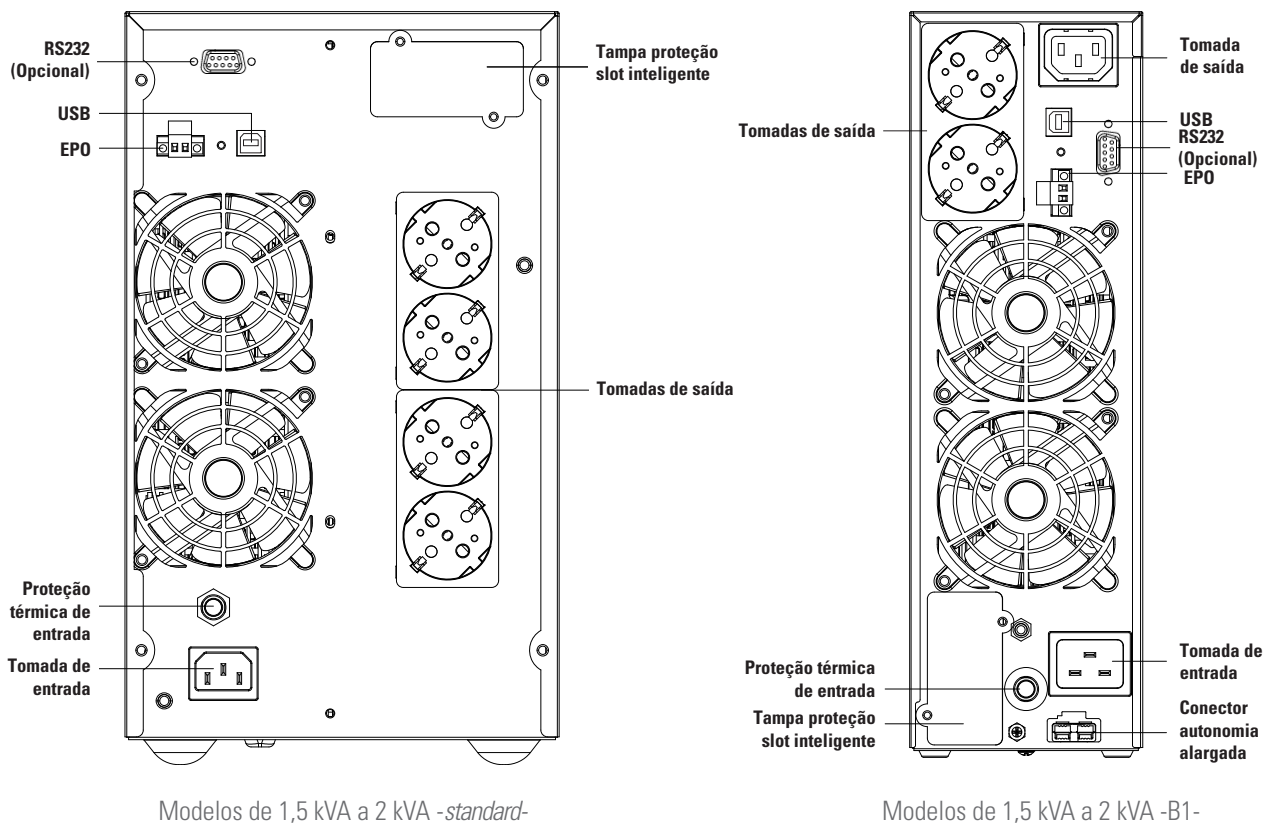
Fig. 7. Vistas posteriores, modelos de 1,5 kVA a 2 kVA com tomadas de saída schuko.
