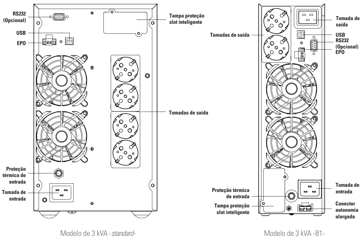
Fig. 8. Vistas posteriores, modelos de 3 kVA com tomadas de saída schuko.
