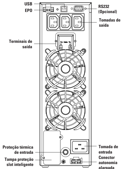
Modelo de 3 kVA -B1-
